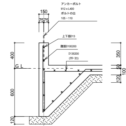
基礎詳細図 1/30
