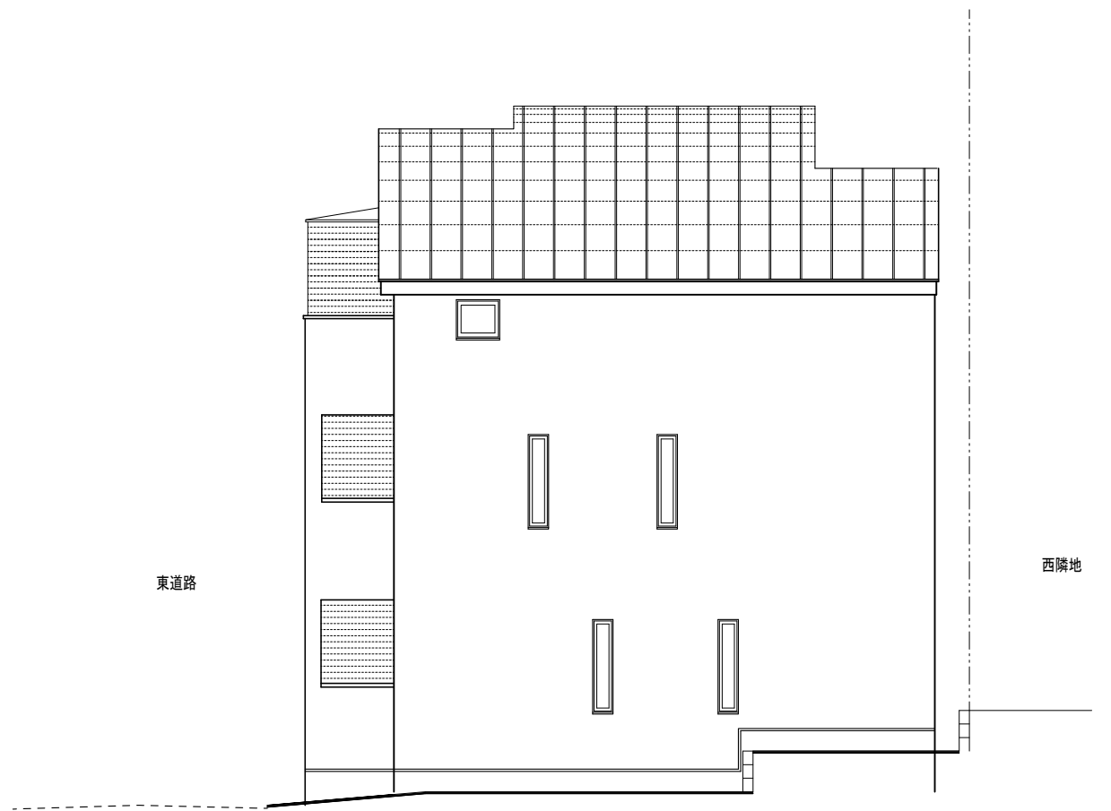
北立面图 1 : 100
