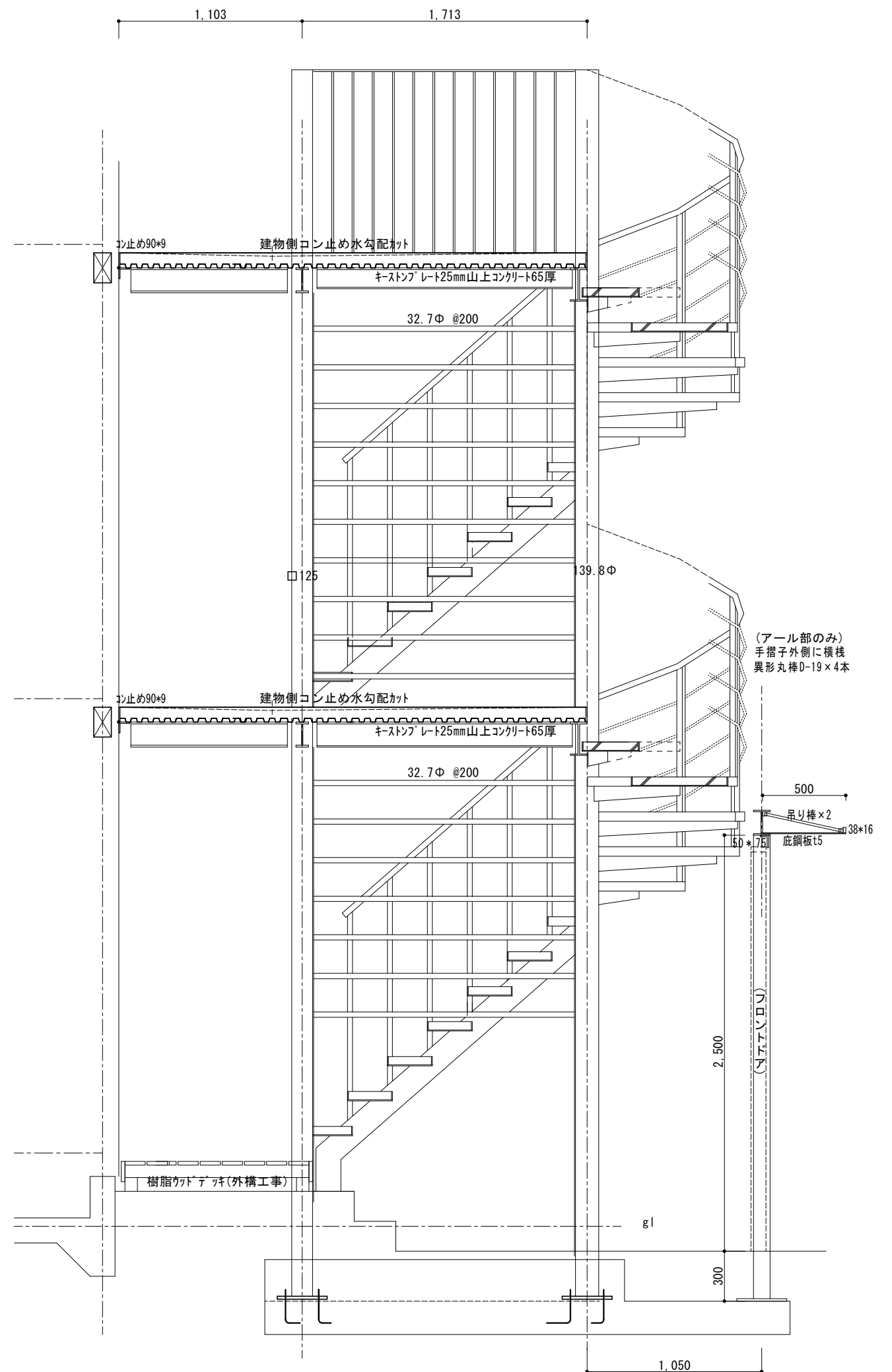
B断面
