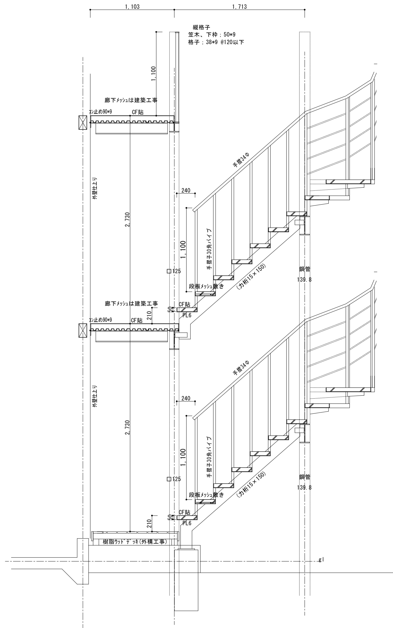
A断面
