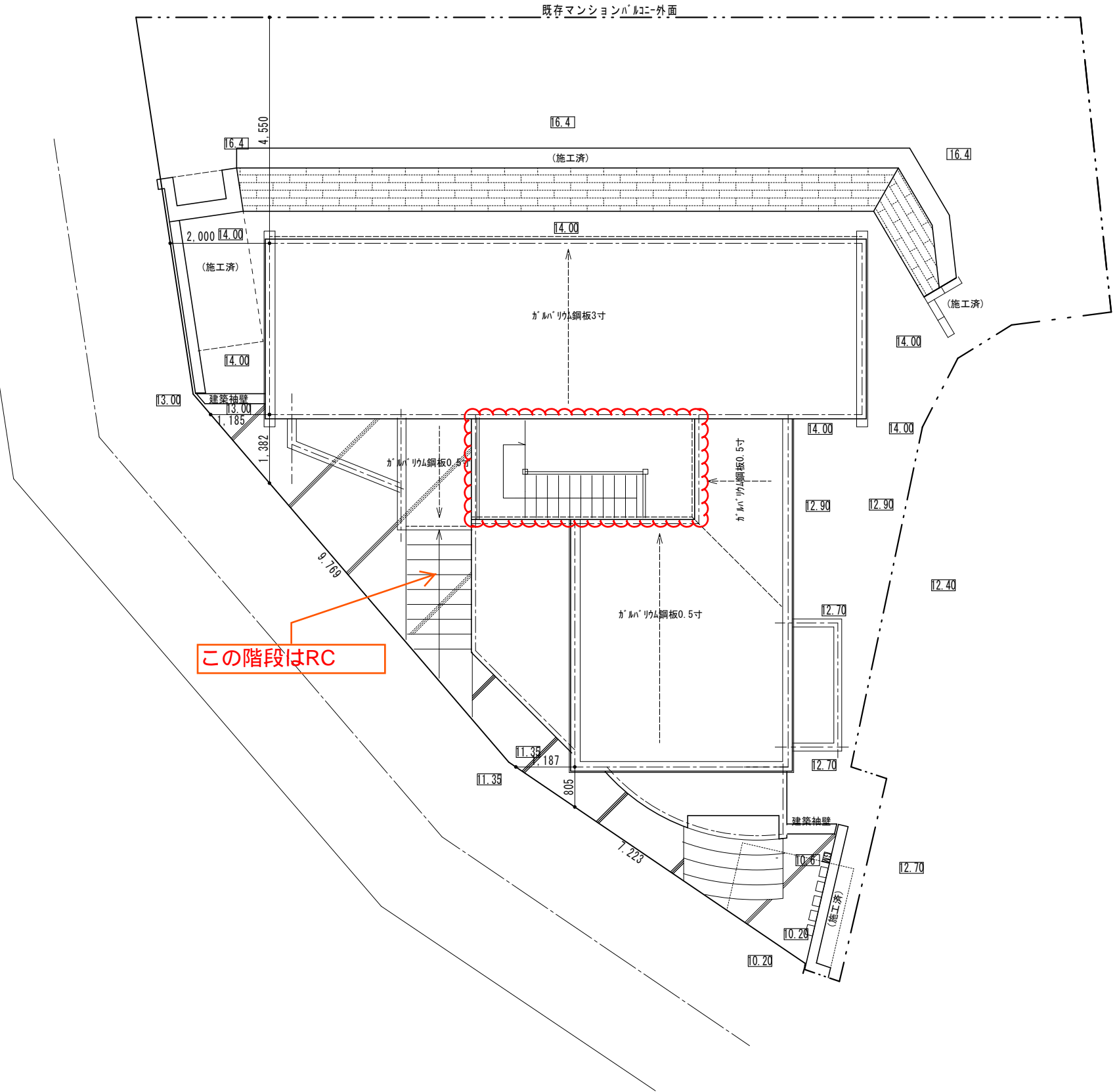
配置図 1 : 100
