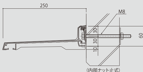
(内部ナット止式)
